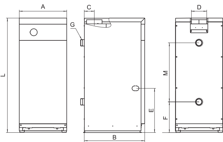
Рисунок 1 Общий вид, габаритные и присоединительные размеры котлов
