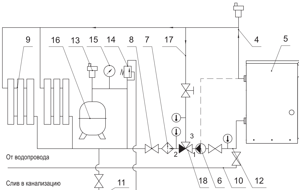
Рисунок 9 Рекомендуемая гидравлическая схема закрытой системы отопления с циркуляционным насосом
