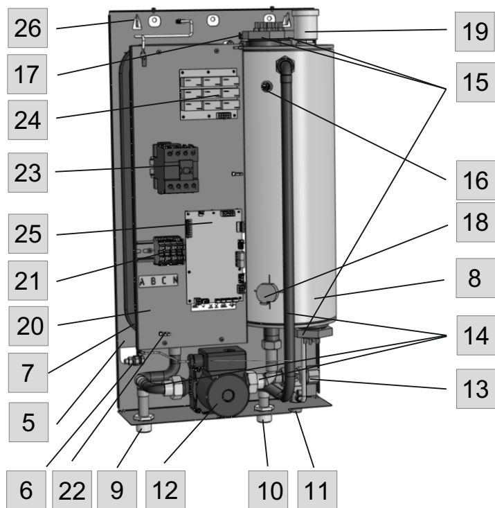
Рисунок 3 Прибор EXPERT со снятыми лицевой панелью и кожухом
