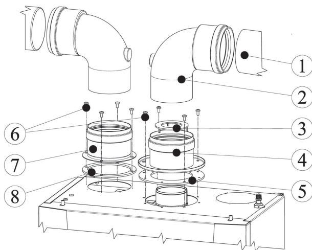
Рис. 7. Пример схемы подключения раздельного дымохода и диафрагмы котел
