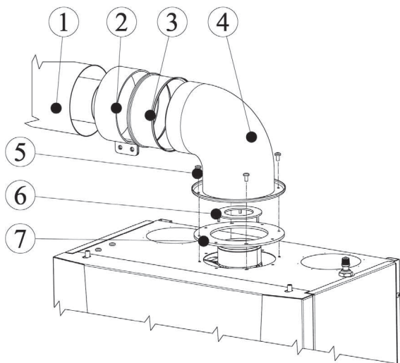
Рис. 6. Пример схемы подключения коаксиального дымохода и дифрغمы котла
