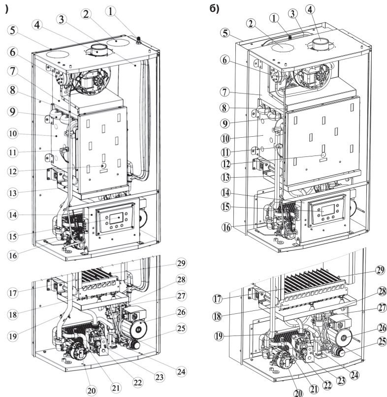
Рис.1. Конструкция котл ) PRIME-V10...24 б) PRIME-V26...32
