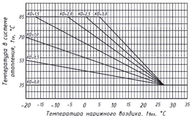
Рис. 8. Кривые н грв
