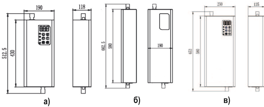
Рисунок 5.1. Габаритные размеры. а) ECO-3, ECO-4,5; б) ECO-6, ECO-7,5, ECO-9, ECO-12, в) ECO-15, ECO-18
