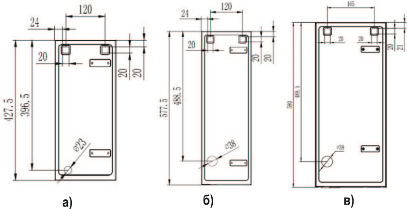
Рисунок 5.2. Монтажные размеры для крепления на стены. Вид с тыльной стороны котла. а) ECO-3, ECO-4,5; б) ECO-6, ECO-7,5, ECO-9, ECO-12; в) ECO-15, ECO-18
